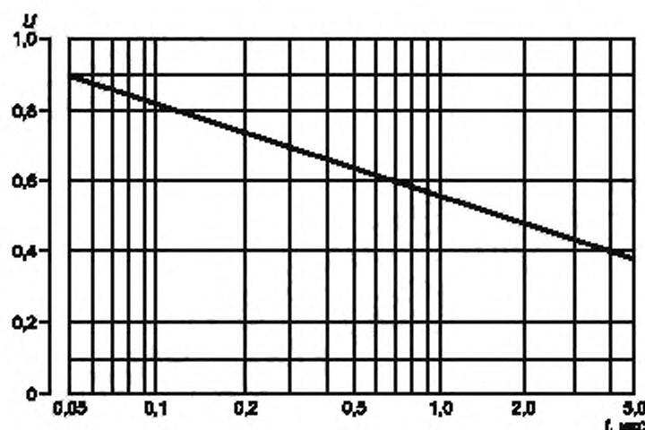
Рисунок 9 — Худший случай распределения напряжений в межвитковой изоляции разнообразных выпных обмоток статора в функции времени нарастания импульса
