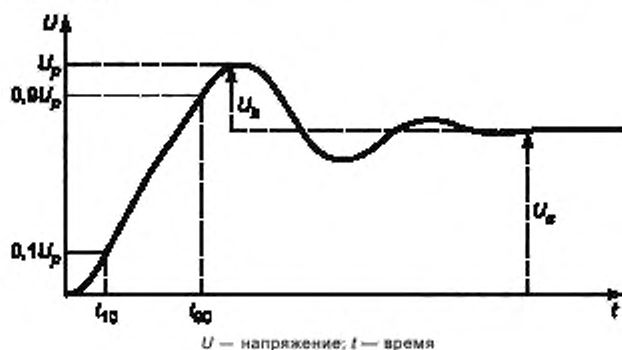
Рисунок 1 — Параметры импульса напряжения
