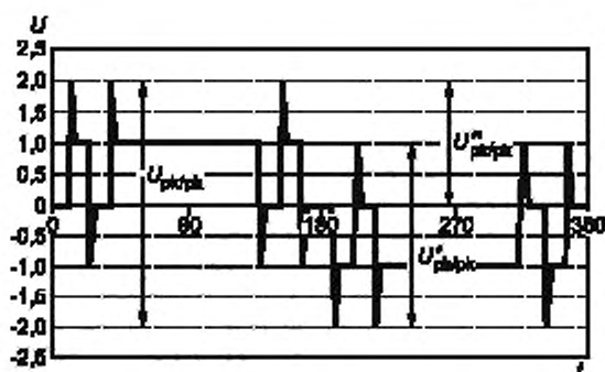
U_{\text{pk/pk}} — межпиковое напряжение основной частоты; U'_{\text{pk/pk}} — межпиковое напряжение на частоте импульсов; U''_{\text{pk/pk}} — скачок напряжения
