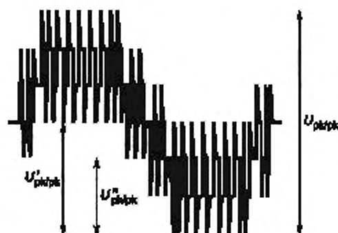
Рисунок 4 — Напряжение на зажимах двигателя при питании от трехуровневого преобразователя
