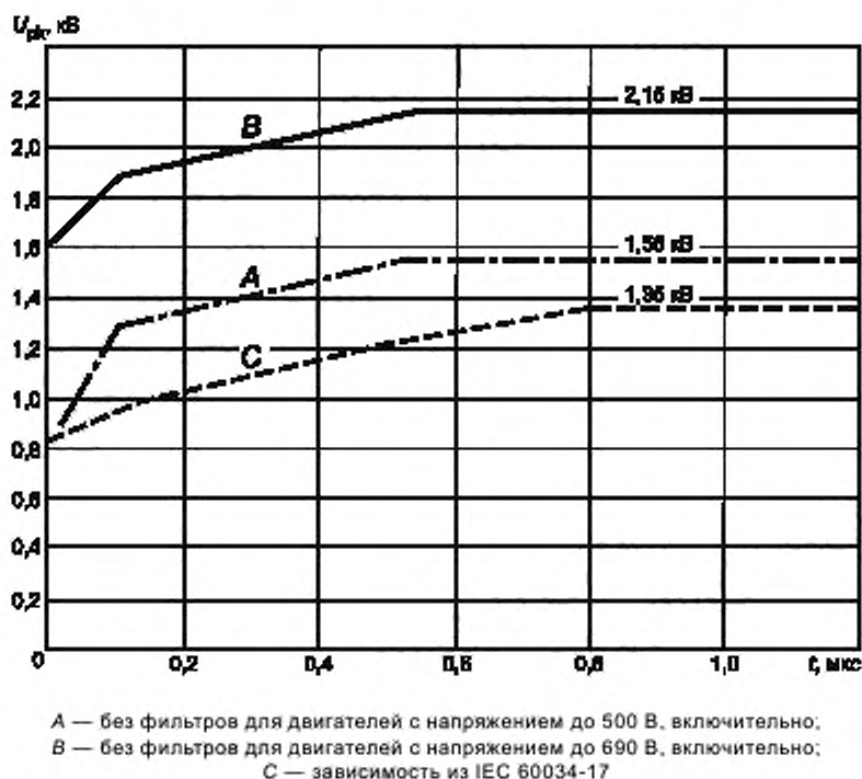
Рисунок А.2 — Граничные кривые импульсного напряжения U_{pk} , приложенного между двумя фазными зажимами двигателя в функции времени нарастания импульса t_r .
