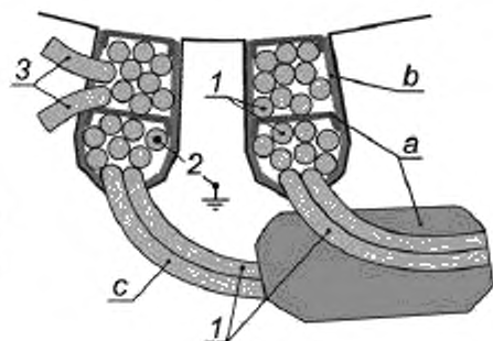
a — изоляция фазы (межкатушечная изоляция); b — лазовая изоляция (от заземленных деталей); c — витковая изоляция; 1 — межфазная изоляция; 2 — изоляция между обмоткой и заземленными частями машины; 3 — межвитковая изоляция
