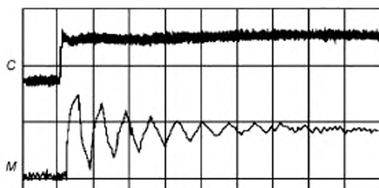
С — напряжение преобразователя; М — напряжение двигателя
