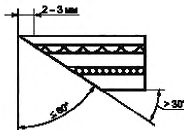
Рисунок А.7 — Факетированный край
