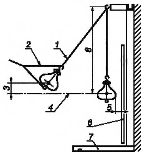
1 — трос; 2 — узел для подъема мешка; 3 — высота падения мешка; 4 — центр образца; 5 — расстояние между образцом и мешком, висющим в свободном состоянии; 6 — испытуемый образец, закрепленный в раме; 7 — опора, 8 — высота подвеса
