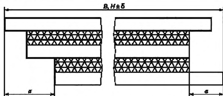
B, H — длина и ширина многослойного стекла; \alpha — смещение листов стекла в многослойном стекле; \delta — допуск (предельное отклонение) на длину и ширину многослойного стекла
