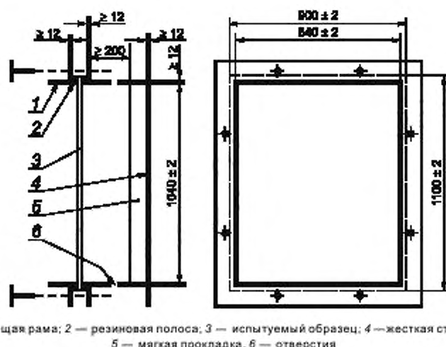
Рисунок 2 — Стальная зажимающая рама
