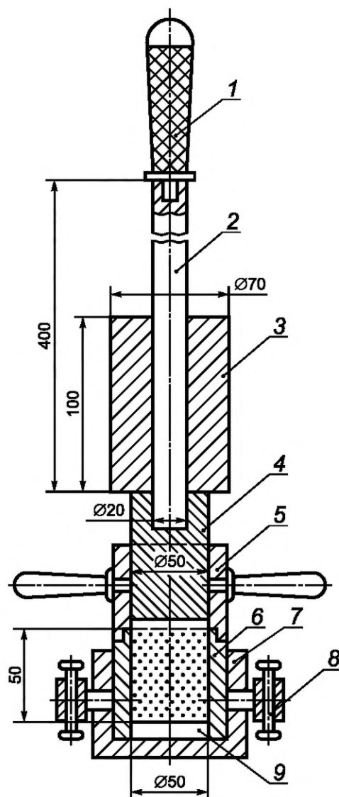
1 — рукоятка; 2 — направляющий стержень; 3 — гиря; 4 — плунжер; 5 — направляющий насадный цилиндр; 6 — разъемный цилиндр; 7 — подстанник; 8 — закрепляющие винты; 9 — металлическая пластинка
