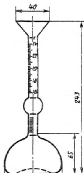
Рисунок 1 — Прибор Ле-Шателье
