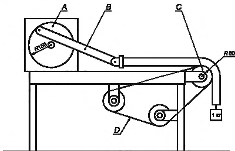
A — кривошипный механизм; B — соединительная тяга; C — ролик; D — абразивная лента
