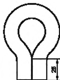
Рисунок 103 — Конфигурация шланга для его замораживания
