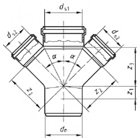
а) Крестовина
