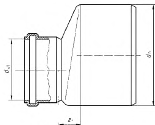
Рисунок 8 – Патрубок переходной
