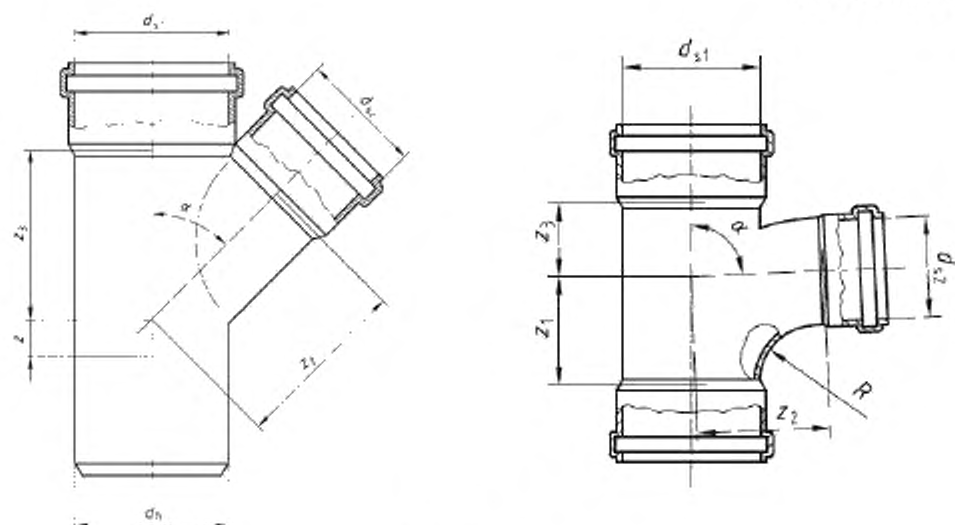
а) Тройник
