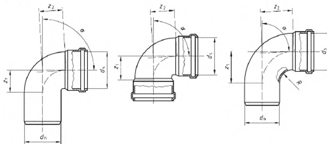
а) Отвод
