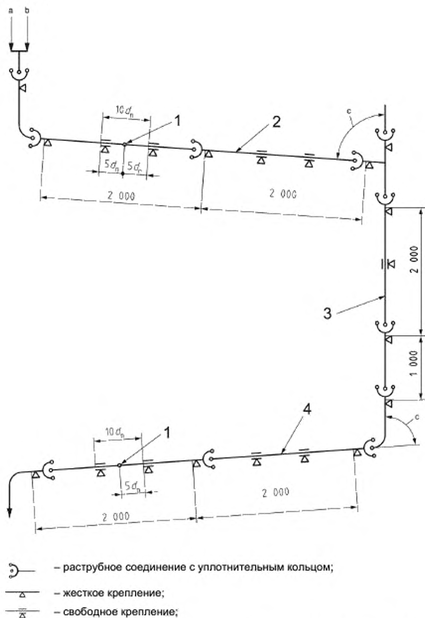
1 — измерение прогиба труб; 2 — трубы d_n = 40 мм или d_n = 50 мм; 3, 4 — трубы 75 \text{ мм} \leq d_n \leq 160 \text{ мм} ; а — подача горячей воды, б — подача холодной воды, с — угол от 85^\circ до 89^\circ
