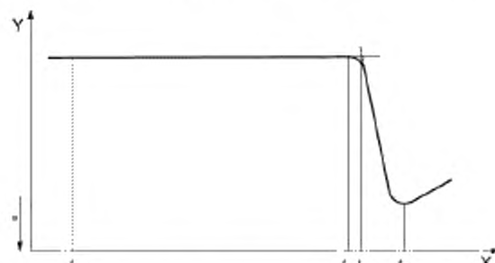
X — время; Y — тепловой поток; а — максимум экзотермы; t_1 — переключение на кислород или воздух (время ноль); t_2 — начало окисления; t_3 — точка определенная методом касательной; t_4 — максимум окисления
