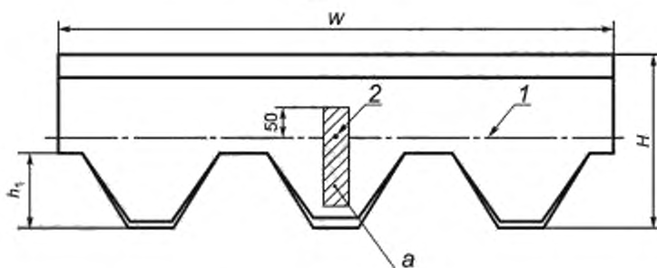
б) Двухслойная черепица
