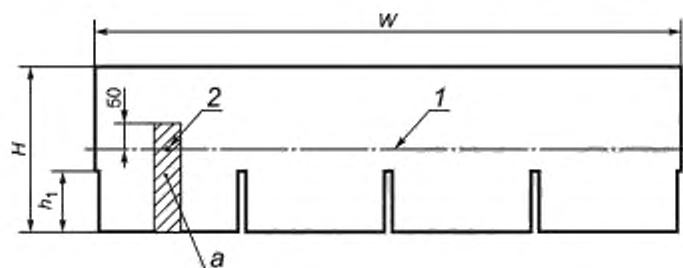
а) Однослойная черепица
