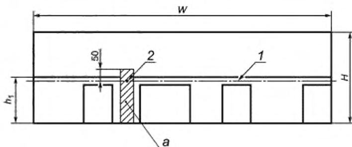
а) Однослойная черепица
