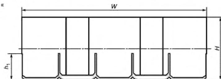
е) — Пример трехслойной черепицы;
