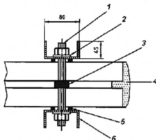
Рисунок Д.2 – Сборный образец-плита в кондукторе для формирования зазора (клеящего шва) – вид спереди
