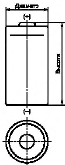
Рисунок 1 — Цилиндрический аккумулятор
