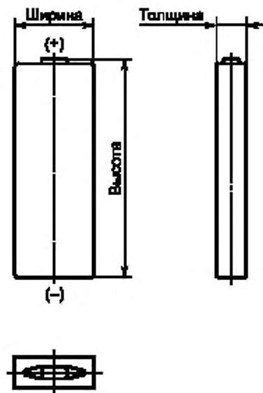
Рисунок 2 — Малогабаритный призматический аккумулятор
