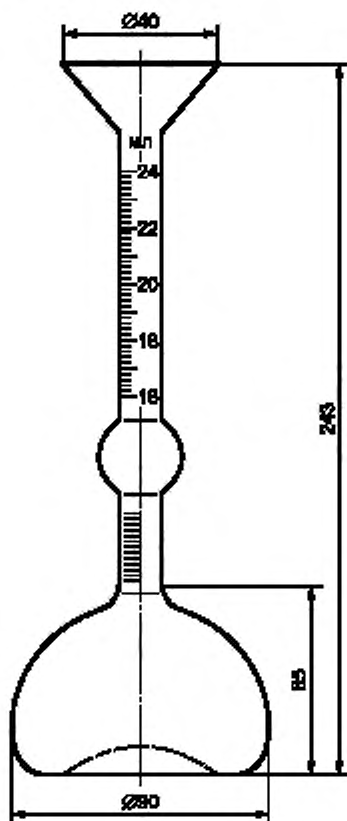
Рисунок 1 — Прибор Ле-Шателье
