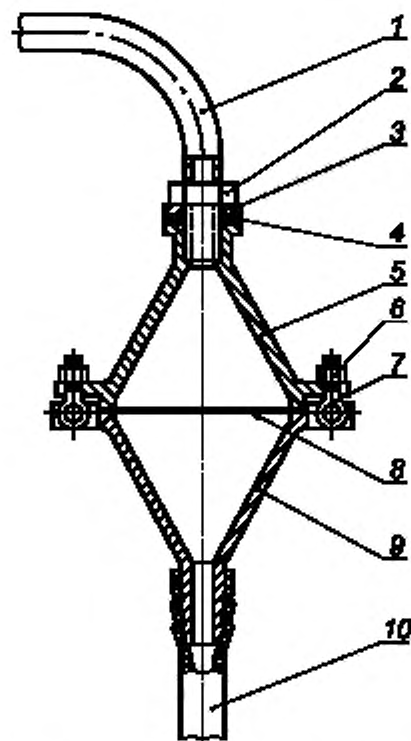
1 — трубка соединительная; 2, 6 — гайка; 3 — шайба; 4 — прокладка; 5, 9 — крышка; 7 — пикт. 8 — фильтр; 10 — трубка резиновая
