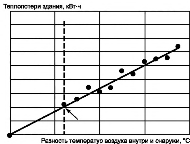
Стрелкой отмечены суммарные тепловыделения в помещениях здания
