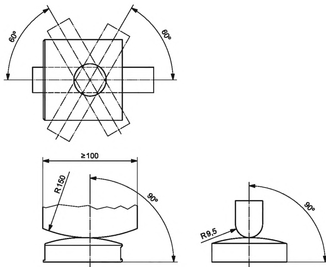
Рисунок 4 — Сжатие пряжки
