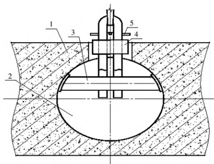
1 – многпустотная плита; 2 – внутренняя полость; 3 – подхватный элемент; 4 – фиксатор; 5 – упор
