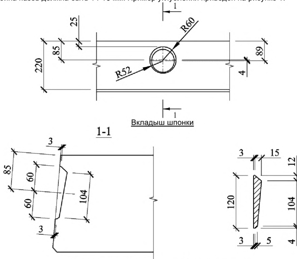
Рисунок 1 – Углубление на боковой поверхности плиты
