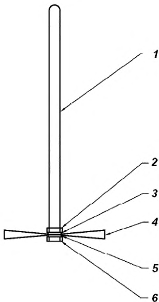
1 – шток мешалки; 2 – гайка; 3 – шайба; 4 – лопасти мешалки; 5 – шайба; 6 – гайка
