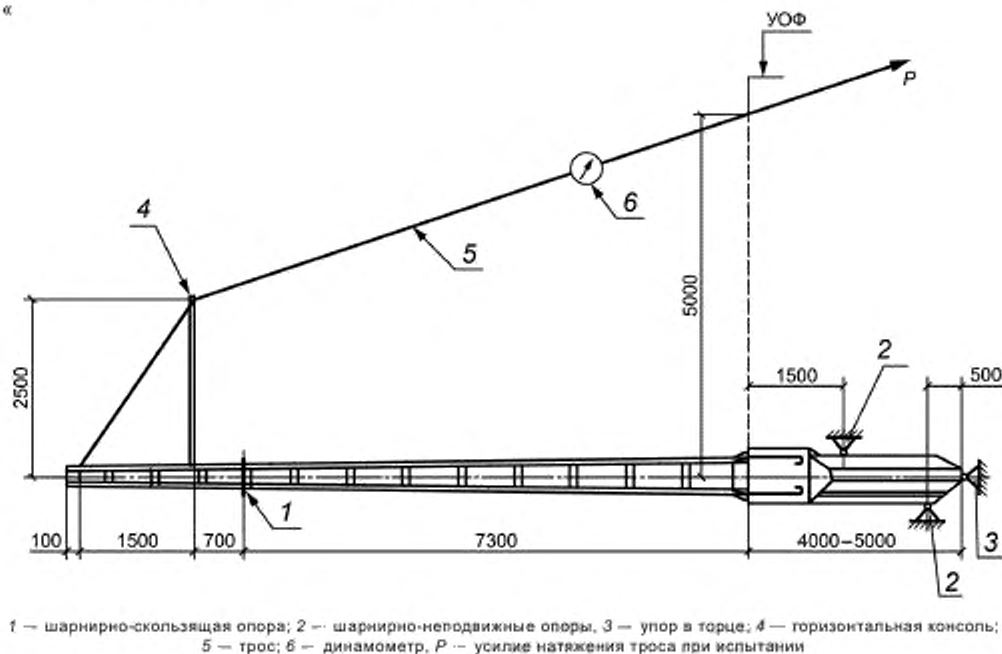
Рисунок В.1 — Схема механических испытаний фундаментов ТСА, ТКА».
