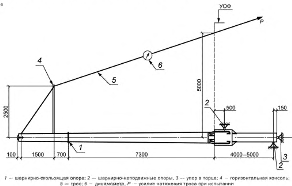
Рисунок Г.1 — Схема механических испытаний фундаментов ФСА».
