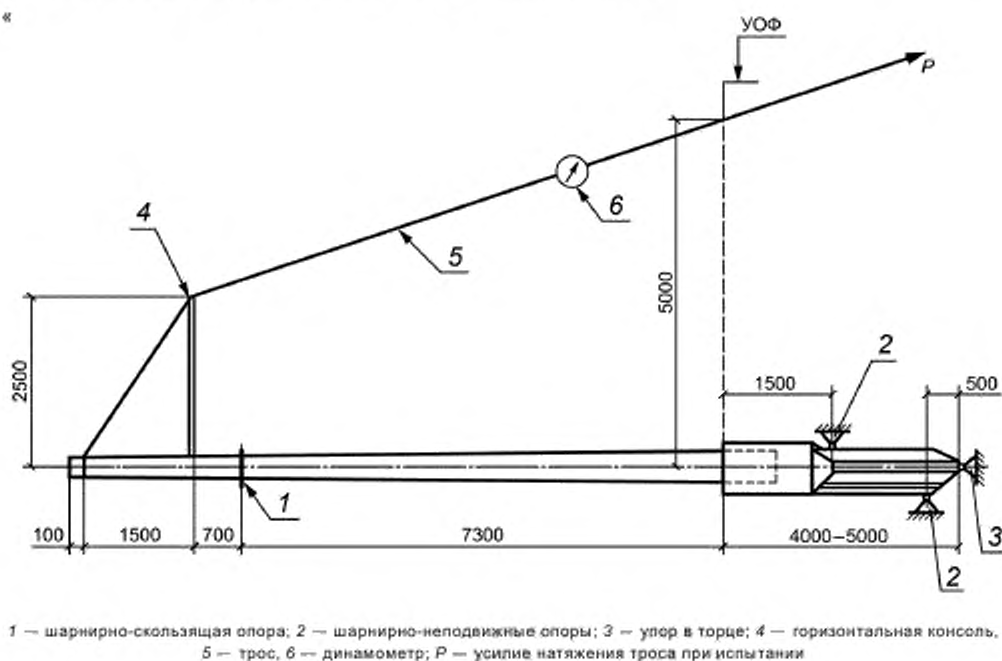
Рисунок Б.1 — Схема механических испытаний фундаментов ТСС».
