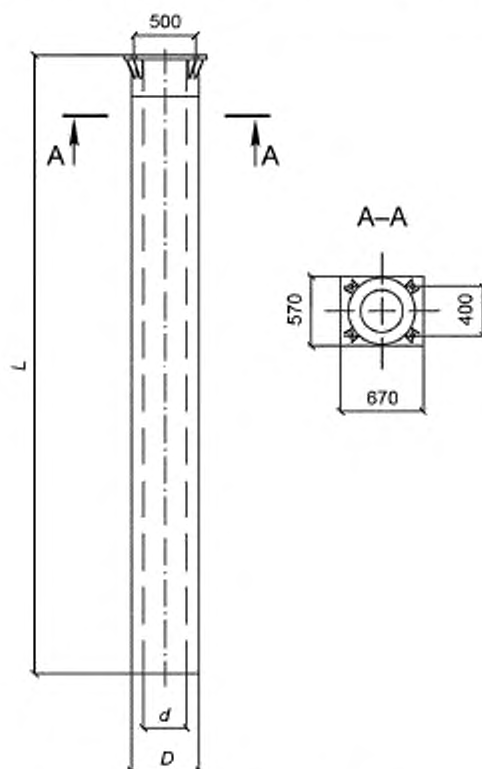
Рисунок 46 — Свая цилиндрическая фланцевая.
