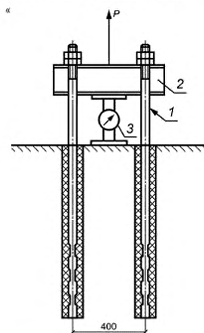
1 — шпилька анкерная; 2 — балка упорная; 3 — домкрат с манометром; P — усилие давления домкрата при испытании
