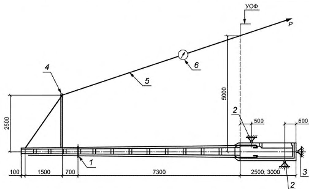
1 — шарнирно-скользящая опора; 2 — шарнирно-неподвижные опоры; 3 — упор в торец; 4 — горизонтальная консоль; 5 — трос; 6 — динамометр; P — усилие натяжения троса при испытании
