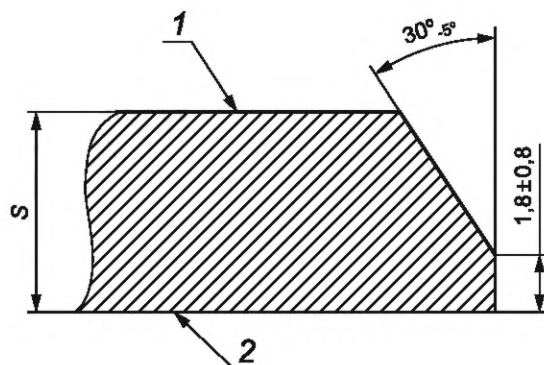
б — При S свыше 3,0 до 15,0 мм включительно
