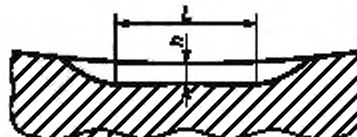
h = (10 \pm 1,5) \% \text{ толщины стенки, но не менее 0,3 мм}
