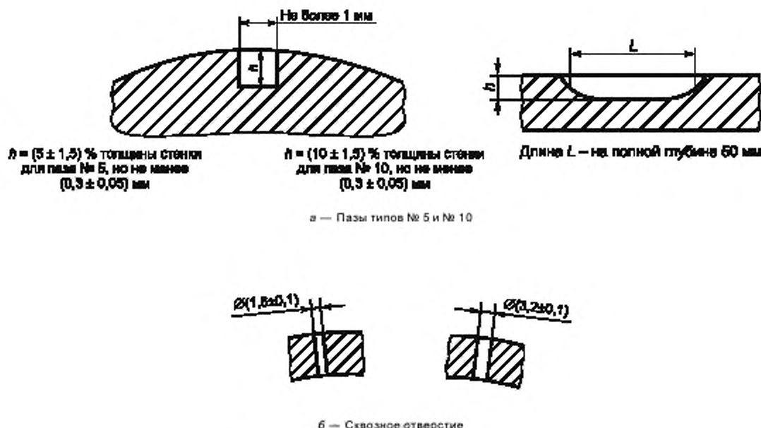
Рисунок В.1 — Виды искусственных дефектов
