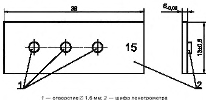
Рисунок Б.1 — Стандартный пластинчатый пенетометр
