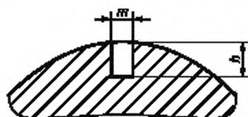
h = (10 \pm 1,5) \% \text{ толщины стенки,} но не менее 0,3 мм
