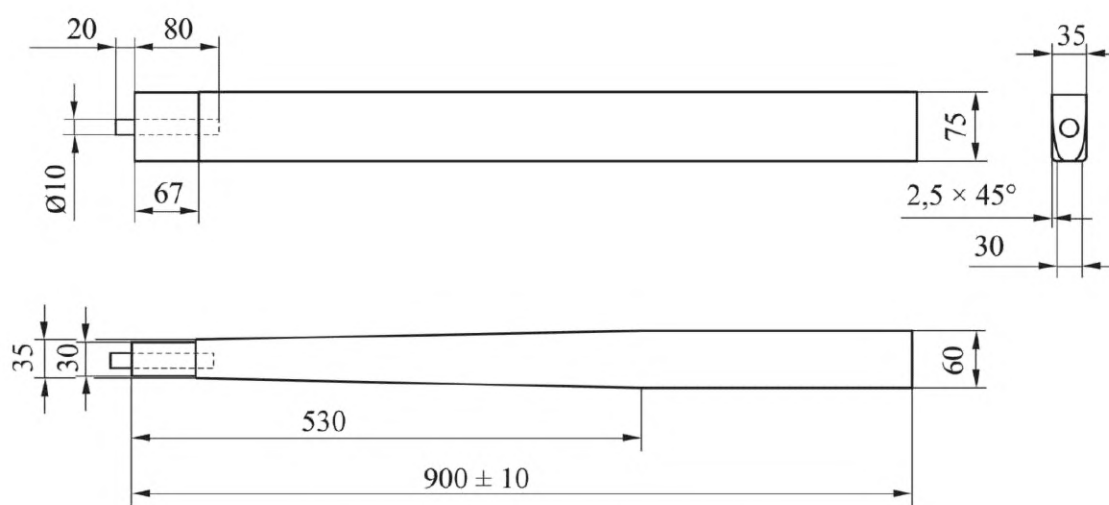
Рисунок 3 – Рукоятка топора (молотка)
