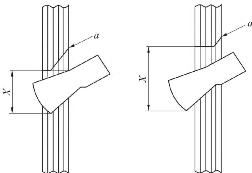
X – длина прорези на обратной стороне образца; a – верхняя часть прорези
