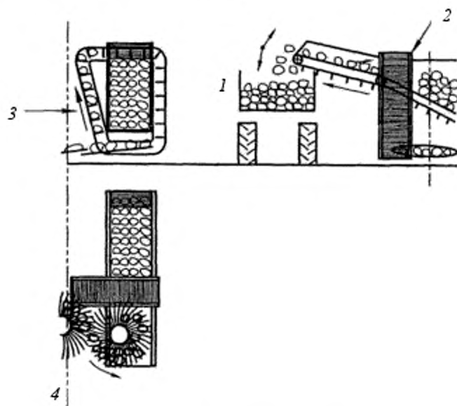
1 – перемещаемый прицеп; 2 – бункер; 3 – лента поднятия корнеплода; 4 – задняя часть машины
