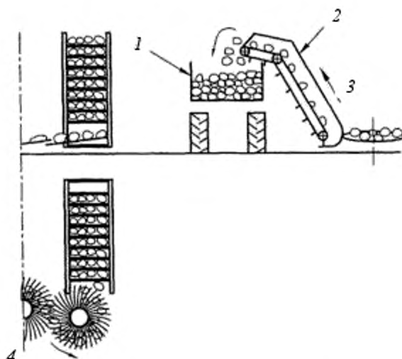
1 – прицеп; 2 – элеватор; 3 – направление загрузки; 4 – задняя часть машины
