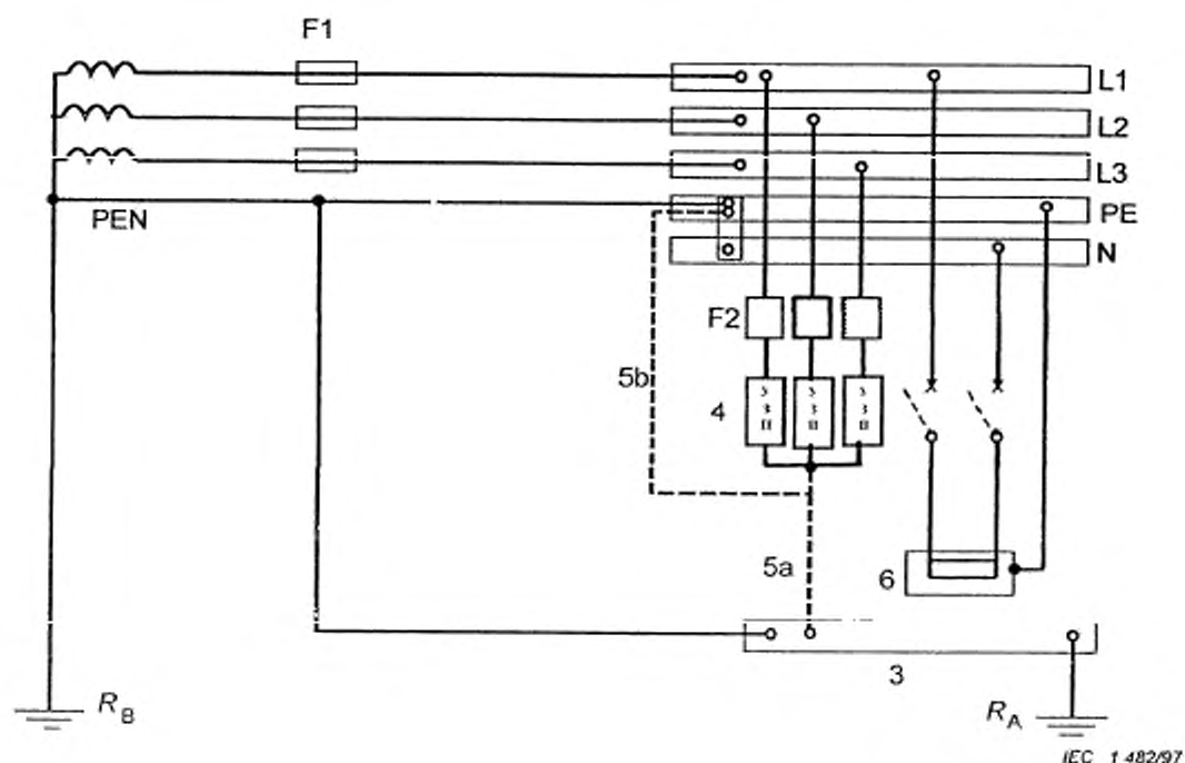
Установка устройств защиты от перенапряжений (УЗП) в системах TN
