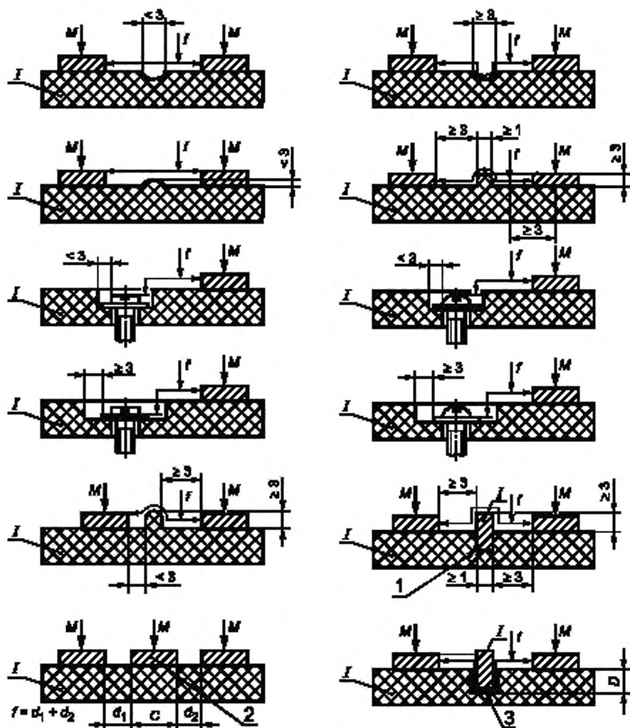
Рисунок 3 – Определение путей утечки (в воздухе)
