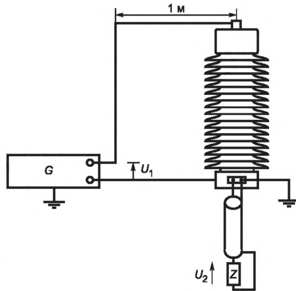
Рисунок 8 — Измерение передаваемых перенапряжений. Типовая испытательная установка
