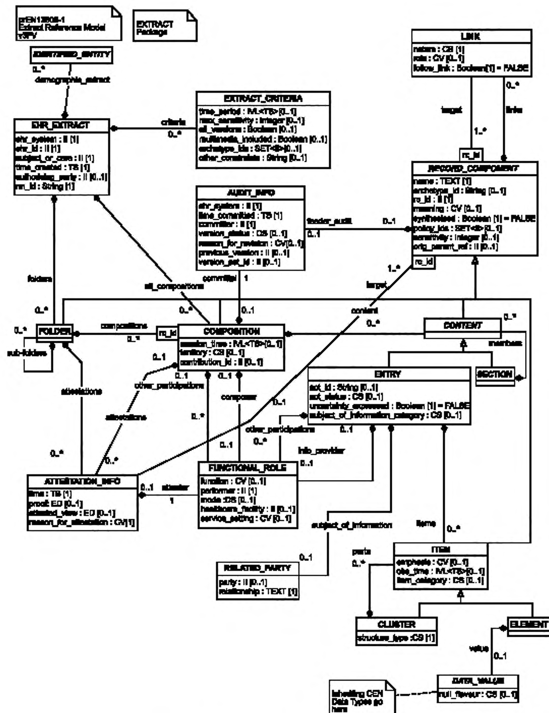
Рисунок 3 — Диаграмма классов UML пакета EXTRACT
