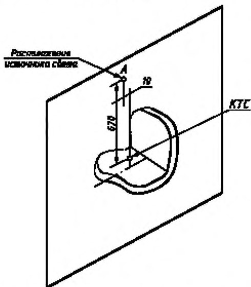
Рисунок 2 — Расположение координат источника света и глаз оператора
