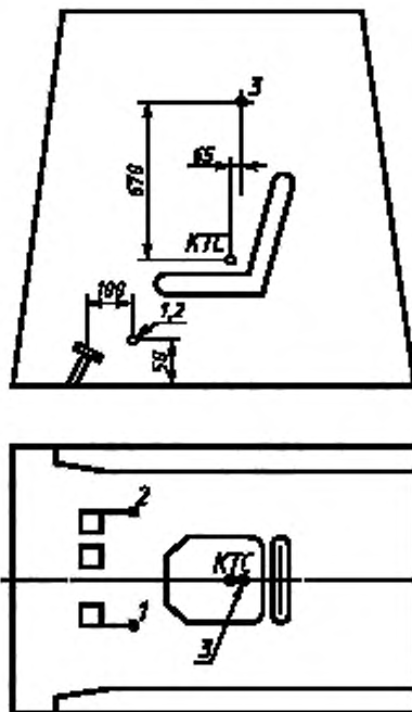
1 3 — точки измерений
