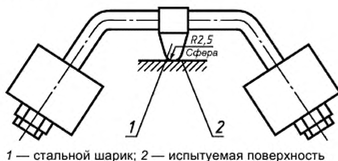
Рисунок 6 — Устройство для испытания вдавливанием шарика
