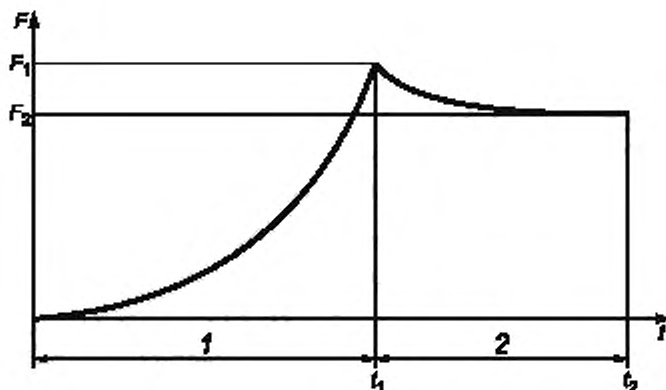
Рисунок А.4 — Динамика релаксации при индентировании
