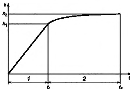
Рисунок А.3 — Ползучесть при индентировании
