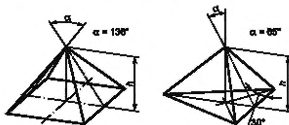
Рисунок А.1 — Форма наконечников для определения НМ
