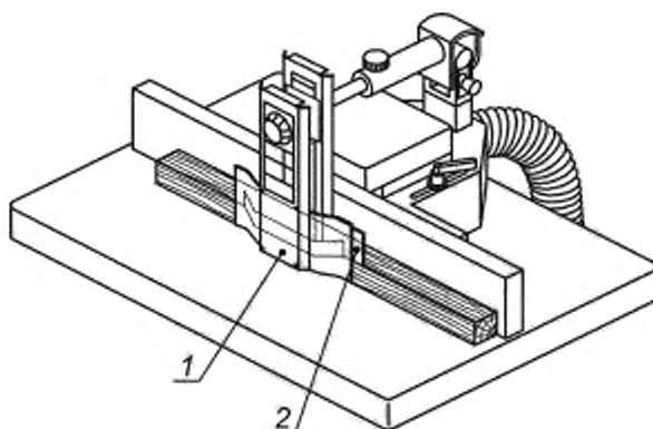
1 — прижимной башмак направляющей линейки; 2 — прижимной башмак стола
