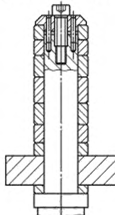
Рисунок 9б) — Пример применения винта, двух штифтов и специального фланца
