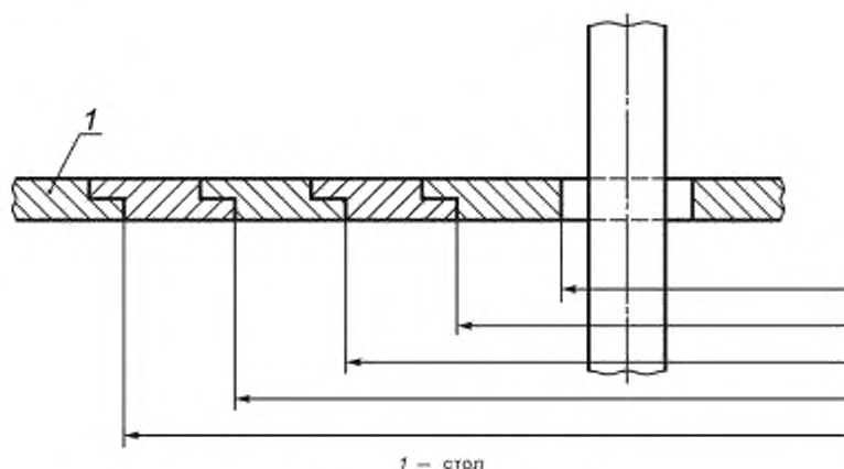
Рисунок 15 — Кольца стола
