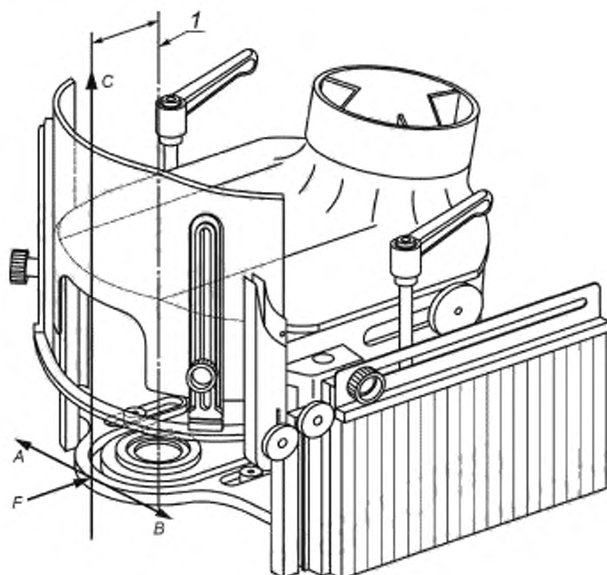
1 — ось шпинделя
