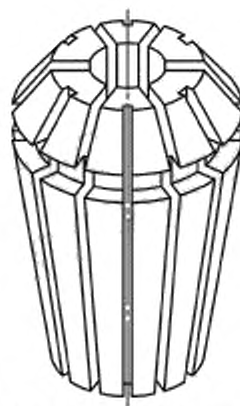
Рисунок 9д) — Зажимная цанга для крепления оправки с закрепленным на ней инструментом
