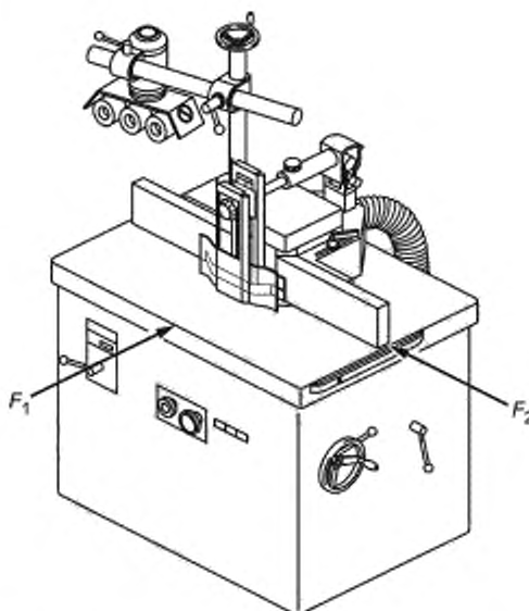
Рисунок С.1 — Испытание на устойчивость передвижных станков
