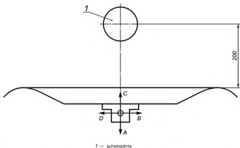
Рисунок В.2 — Направление, точка приложения силы и измерения при испытании на устойчивость прижимного башмака направляющей линейки (вид сверху)
