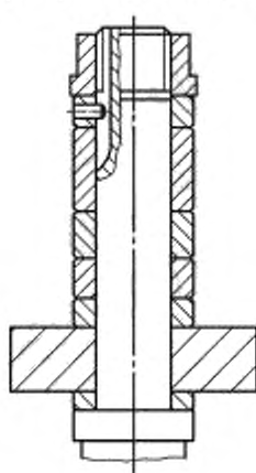
Рисунок 9а) — Пример применения фиксирующего штифта в шпиндельном кольце
