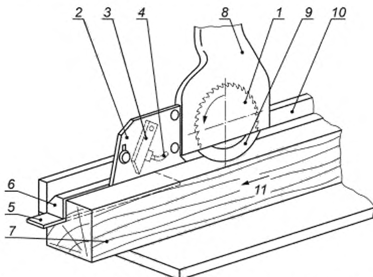
1 — дисковая пила; 2 — отделитель штапика от заготовки; 3 — противовыбрасывающее устройство (планка); 4 — прижимное устройство; 5 — направляющий паз для отрезаемого штапика; 6 — отрезанный штапик; 7 — обрабатываемая заготовка; 8 — неподвижное защитное ограждение дисковой пилы; 9 — автоматически регулируемое по высоте ограждение режущей части дисковой пилы; 10 — направляющая линейка; 11 — направление подачи
