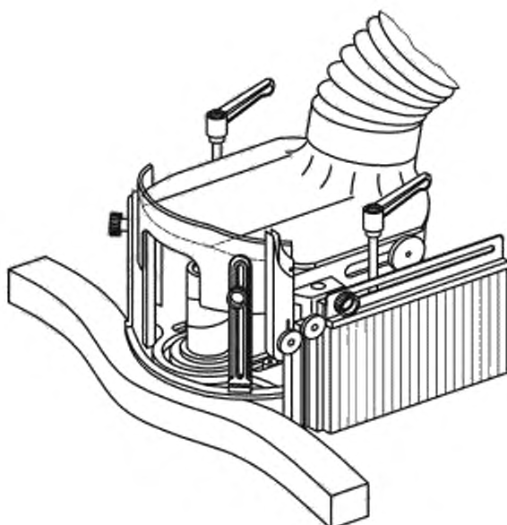
Рисунок 2 — Пример криволинейного фрезерования
