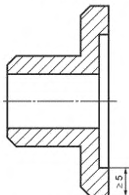
Рисунок 10 — Фланец для крепления дисковой пилы
