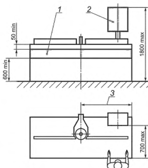
1 — полоса расположения органов управления; 2 — неподвижный пульт управления; 3 — область расположения пульта управления
