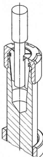
Рисунок 9с) — Пример применения сменных прижимных втулок-вкладышей для крепления оправки с закрепленным на ней инструментом
