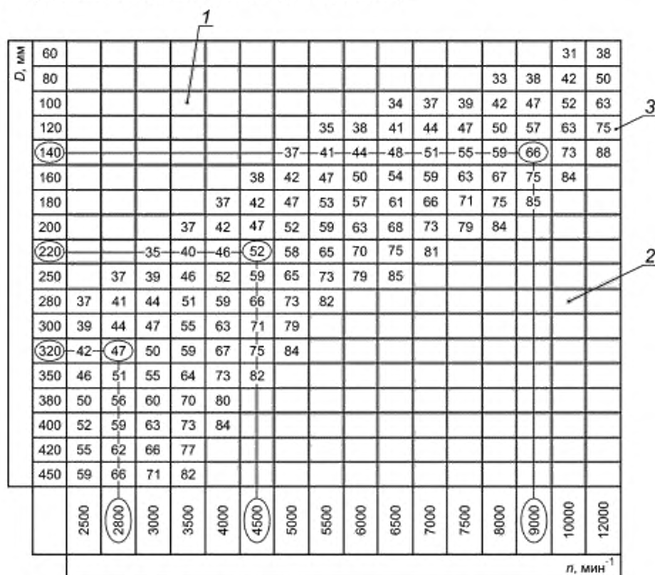
1 — зона низких скоростей резания — плохие условия обработки; 2 — зона чрезмерно высоких скоростей, приводящих к разрушению инструмента и создающих опасность травмирования оператора; 3 — зоны рекомендуемой скорости резания; D — наружный диаметр инструмента (мм), n — частота вращения шпинделя инструмента, мин⁻¹
