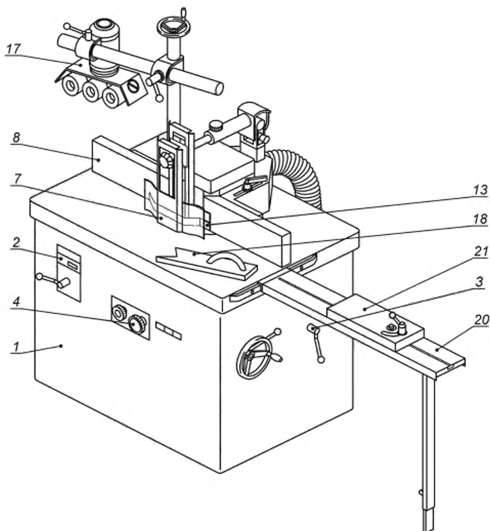
Рисунок 6а) — Пример фрезерного станка, оборудованного для прямолинейной обработки
