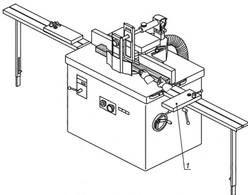
1 — конечный упор для предотвращения отдачи
