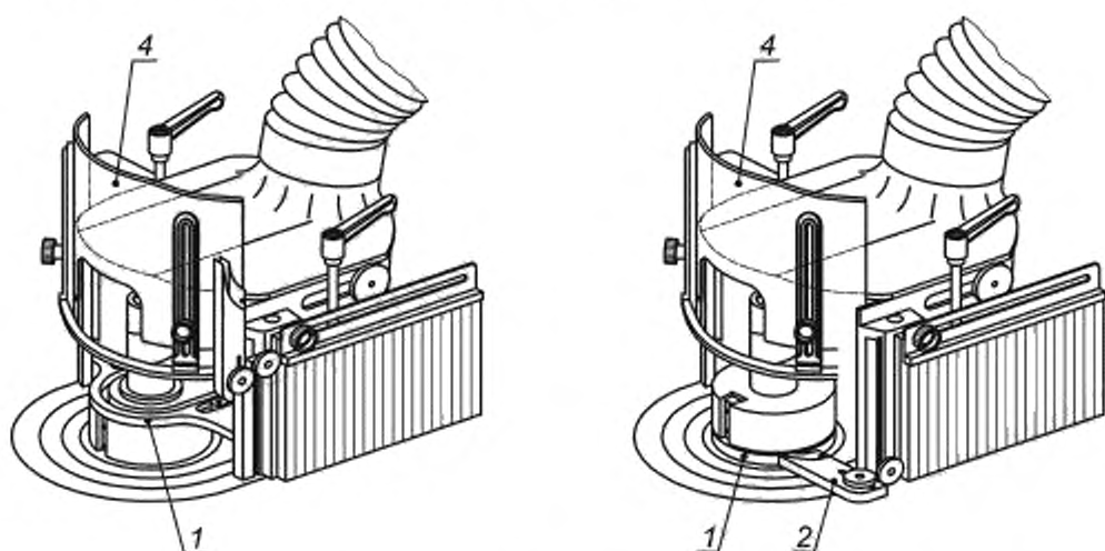
1 — полукруглая направляющая (направляющее кольцо); 2 — приспособления для крепления заготовки с шаблоном; 3 — копирующее кольцо (наружное кольцо шарикоподшипника); 4 — перемещаемое защитное ограждение (перемещаемый щиток)
