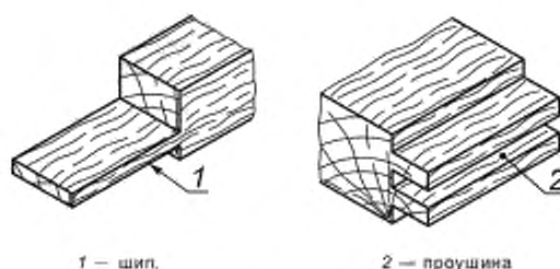
Рисунок 3 — Пример обработанной заготовки с шипом/проушиной
