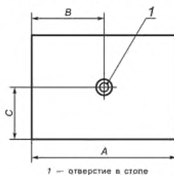
1 — отверстие в столе Рисунок 14 — Основные размеры стола
