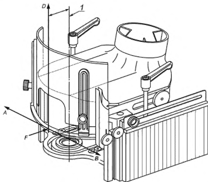
1 - ось шпинделя
