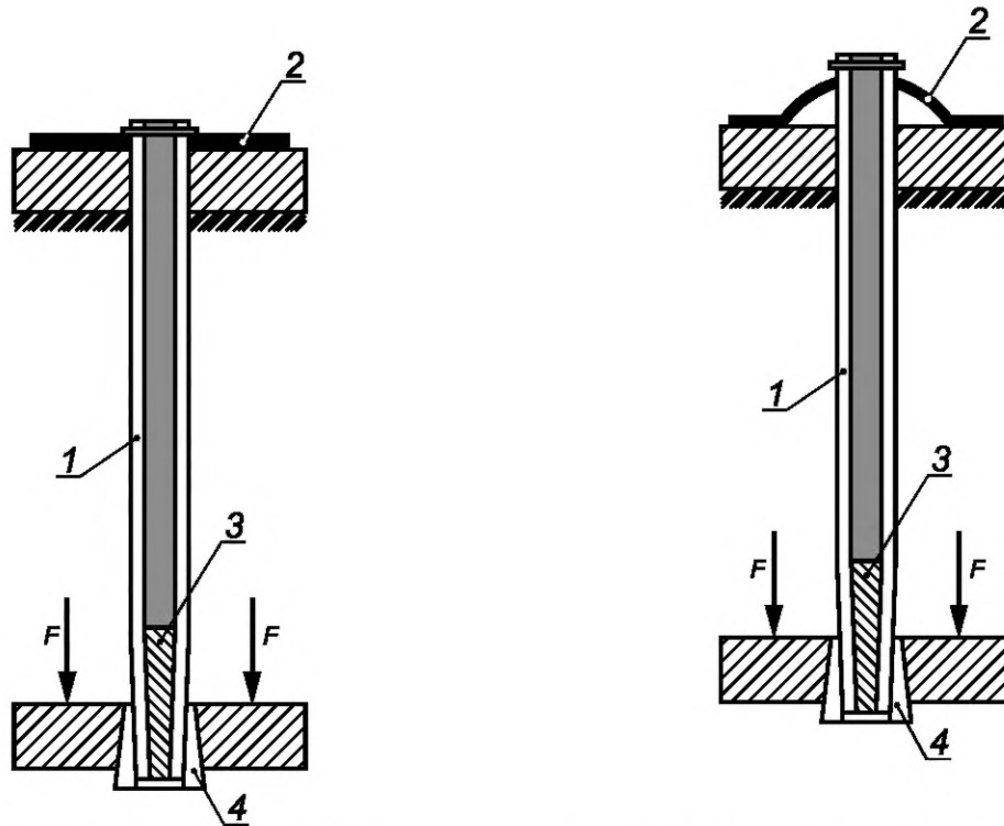
а) Стержень анкера на одинарный срез
