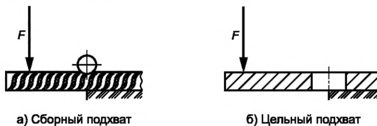
Рисунок 3 — Схема нагружения выпуска подхвата
