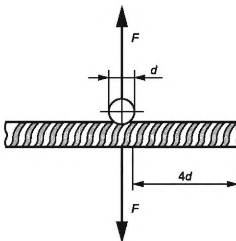
Рисунок 3 — Схема нагружения крестообразных соединений фрагмента сборного подхвата».
