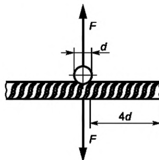
Рисунок 4 — Схема нагружения крестообразных соединений фрагмента сборного подхвата
