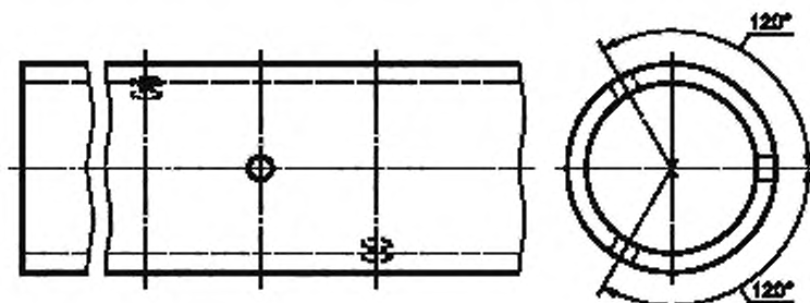
Рисунок Г.1 — Эталонный образец с тремя отверстиями
