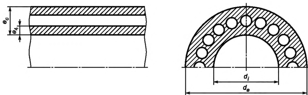
б) Тип А1 (с продольными полыми секциями)
