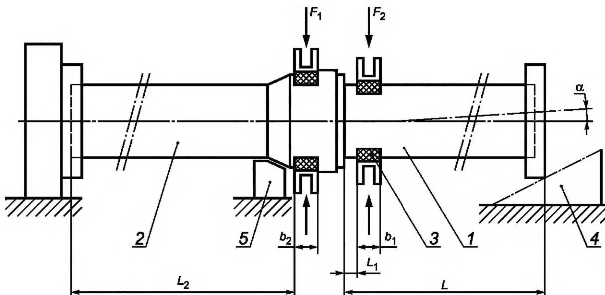
1 — труба; 2 — труба или фасонная часть с раструбом L_2 \geq 1000 мм; 3 — захваты; 4 — регулируемая опора для создания осевого смещения; 5 — фиксатор раструба
