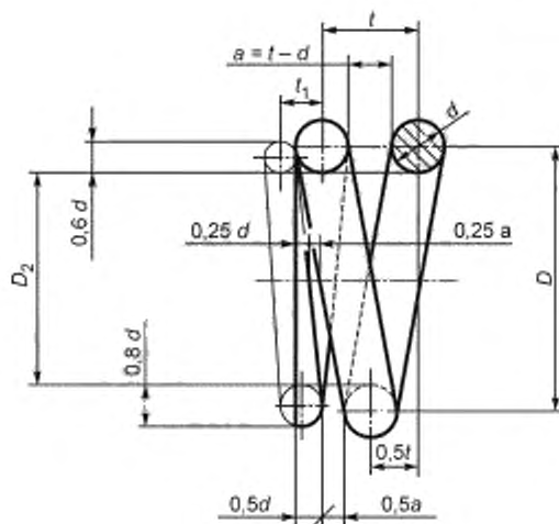
Рисунок В.3 — Крайний виток пружины сжатия с конусообразной формой оттяжки концов с поджатием на \frac{3}{4}d дуги окружности
