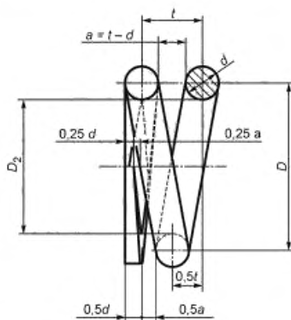
Рисунок В.4 — Крайний виток пружины сжатия с клинообразной формой оттяжки концов с поджатием на \frac{3}{4}d дуги окружности.
