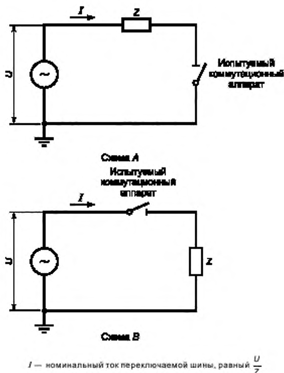
Рисунок 8 — Испытательные цепи для испытаний на включение и отключение уравнивающего тока
