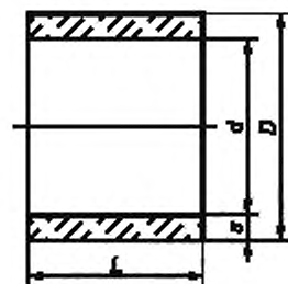
Рисунок 2 — Безнапорная муфта
