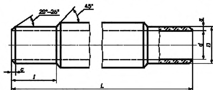
Рисунок 3 — Напорная труба
