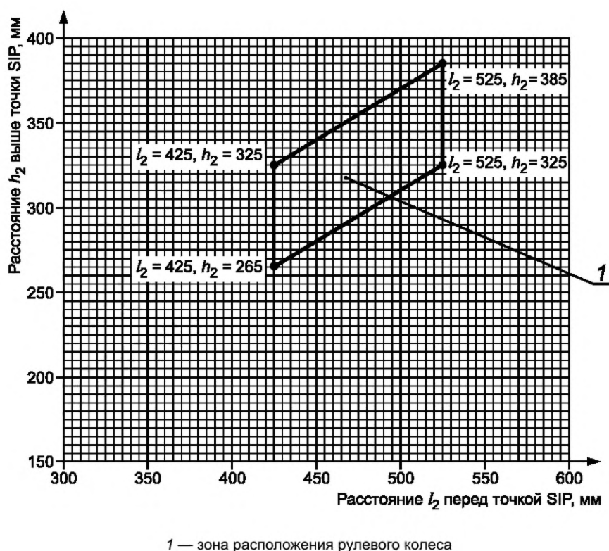
Рисунок 4 — Расположение рулевого колеса относительно точки SIP
