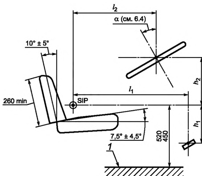
Рисунок 1 — Расположение сиденья оператора, вид сбоку
