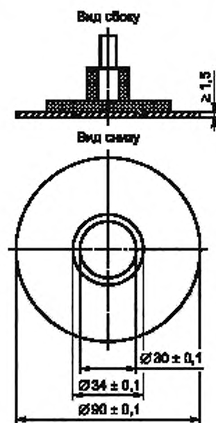
Рисунок 5 — Датчик для измерения поля
