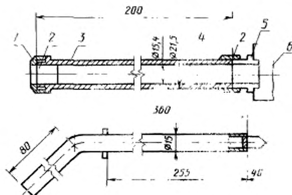
Приспособление для создания и введения искр в выпускную систему двигателя
