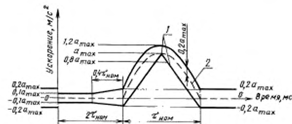
1 — пределы отклонений; 2 — номинальный пробег; a_{\max} — пиковое ускорение удара; t_{\text{ном}} — длительность ударного импульса
