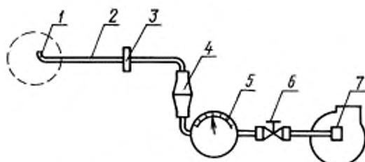
Заборное устройство
